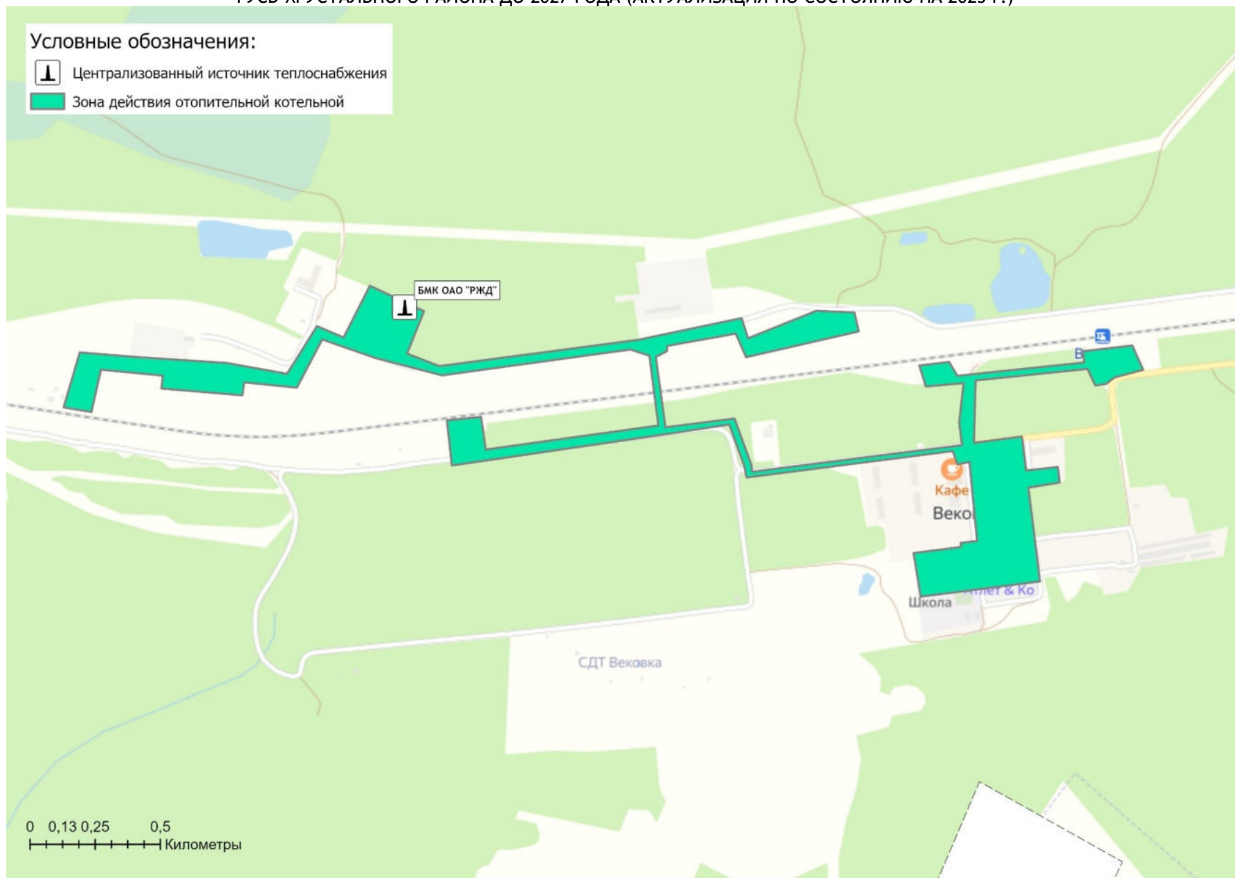
Рисунок 1.4.1 - Зона действия производственно-отопительной котельной на территории ст. Веовка
