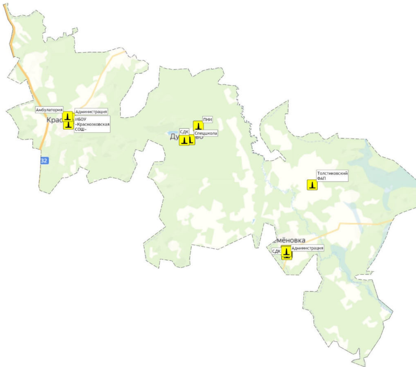
Рисунок 1.2.1 - Расположение ведомственных индивидуальных котельных на территории муниципального образования пос. Красное Эхо (сельское поселение)
