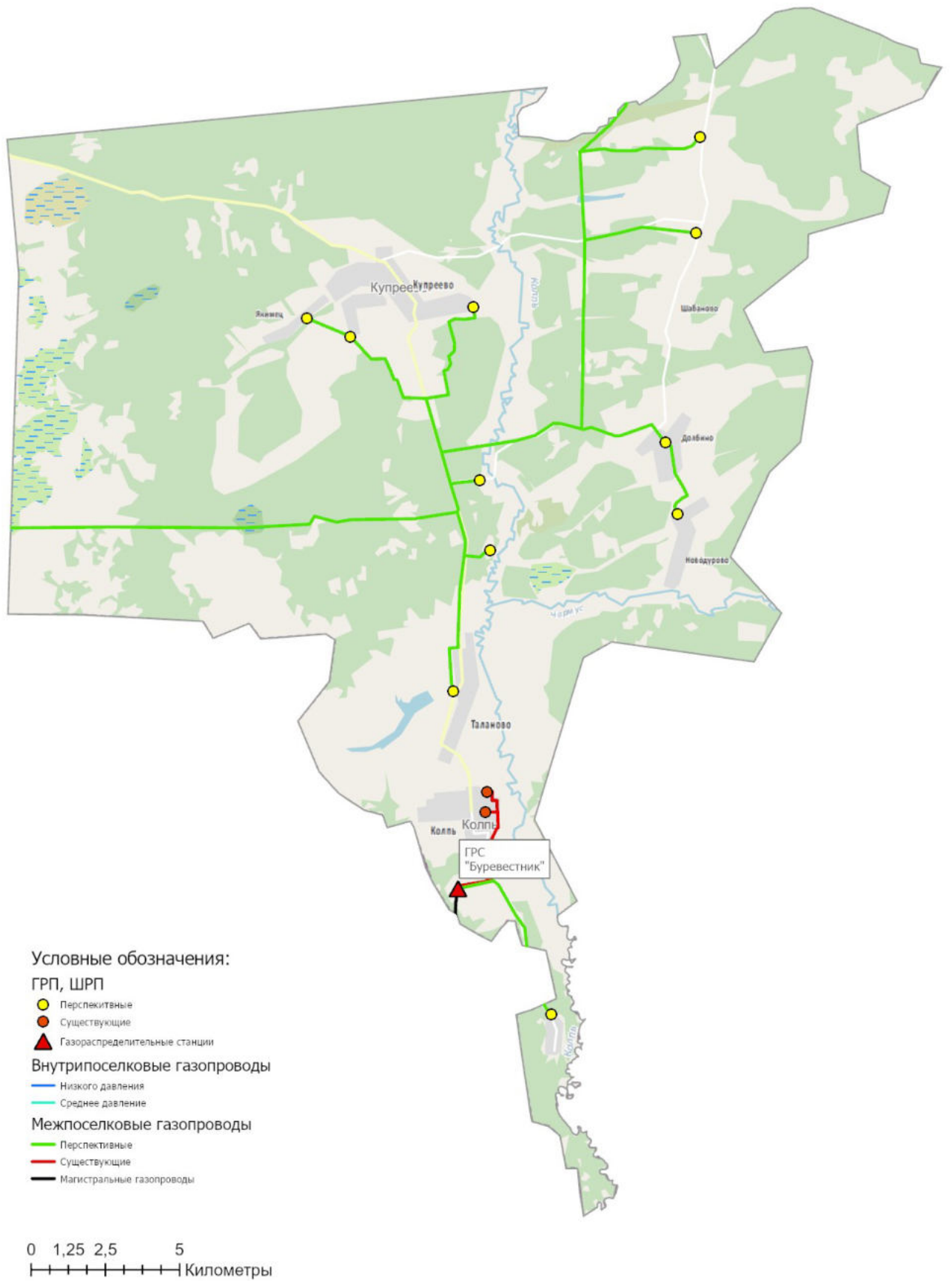
Рисунок 10.6 - Перспективная схема газификации территории муниципального образования
